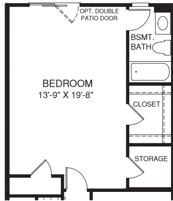
OPT. BEDROOM
