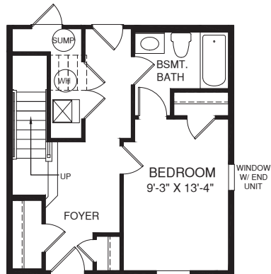
OPT. BEDROOM
