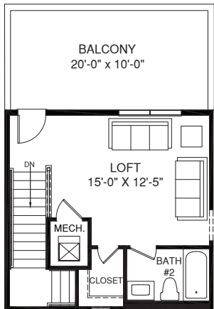
OPT. LOFT
