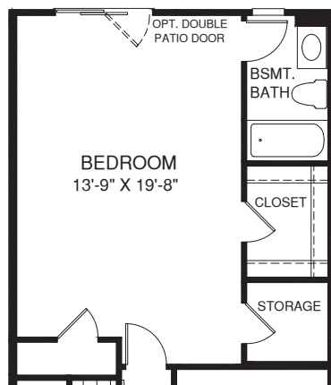
OPT. BEDROOM
