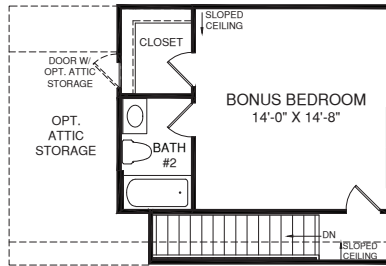
OPTIONAL UPPER LEVEL
